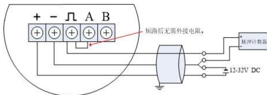
ZRVTD01 显示型信号处理电路接线（脉冲输出）
